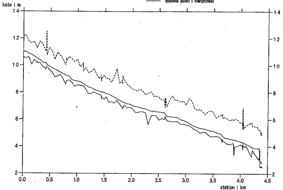
Figur 3.2. Seerdrup å. Længdeprofil med angivelse af terræn, opmålt vandspejl og vandløbsbund. (Seerdrup å. Stream profile, water level and bank elevation.)
